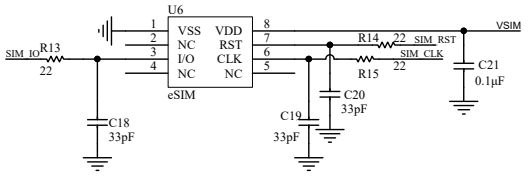
eSIM卡
