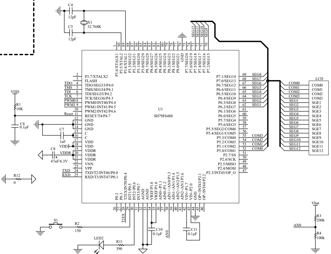
MCU
