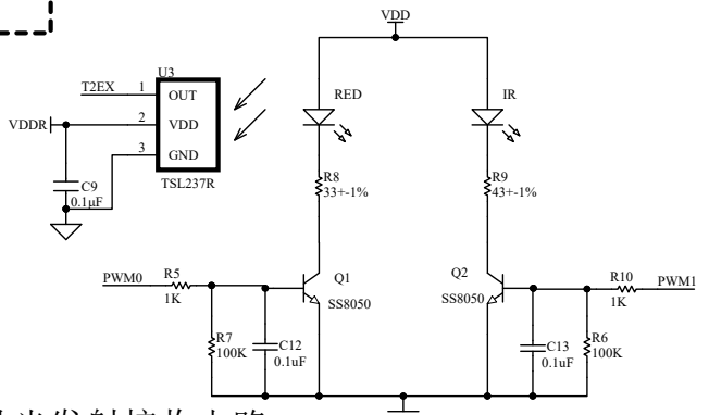
红光红外光发射接收电路
